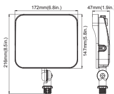
15W&27W(Knuckle Mount)
