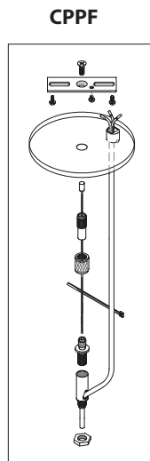
Cord Pendant (Power Feed Capable)
