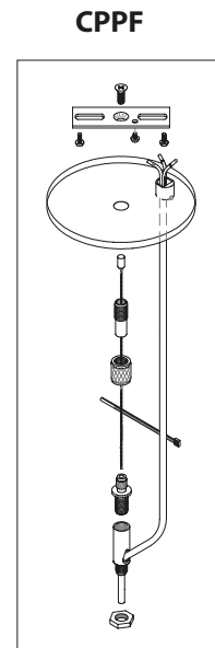
Cord Pendant (Power Feed Capable)
